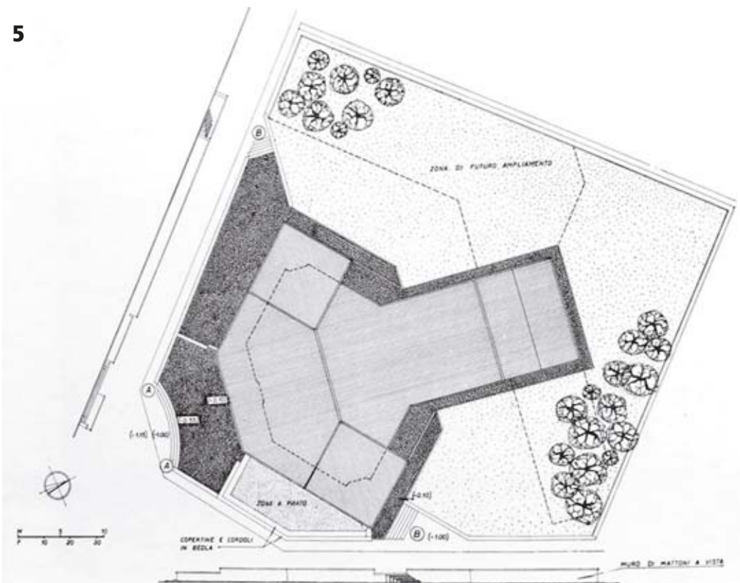
Foto 1 Studio planimetrico del centro comunitario
